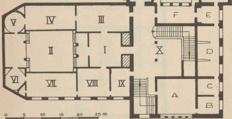
1. OBERGESCHOSS.
